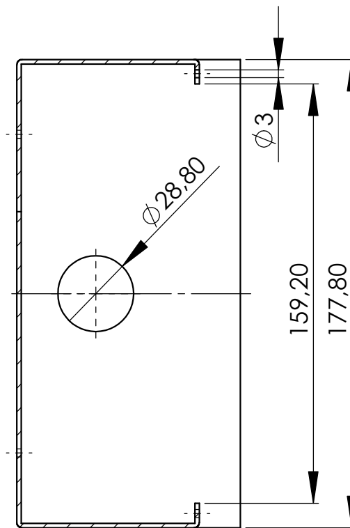
B-B (1 : 2)
